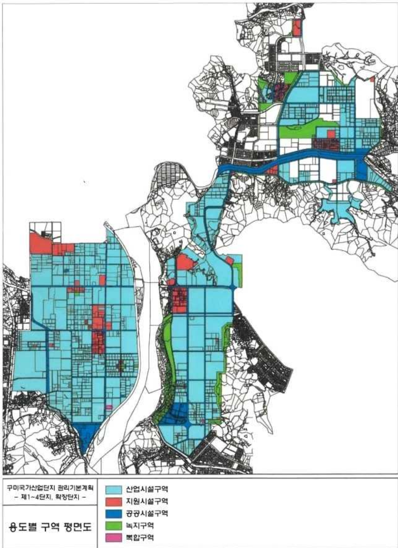
(별첨#1) 구미국가산업단지 용도별구역 평면도(구미국가 제1~4단지, 확장단지)
